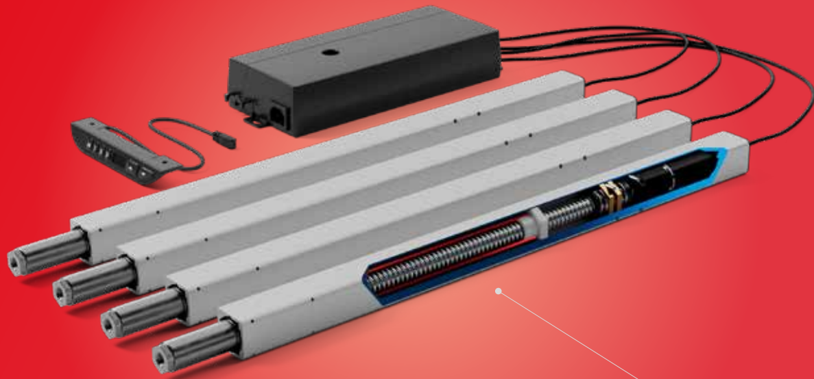
Spindelhubsystem
