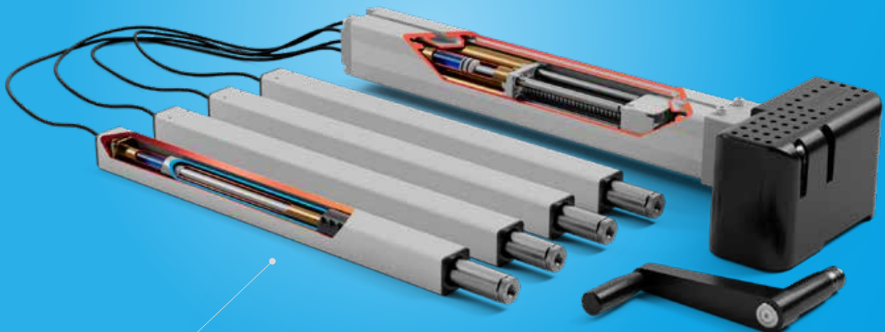
Hydraulikhubsystem
