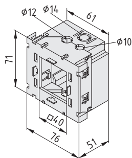
Einbaudose K76 M45 1-fach
