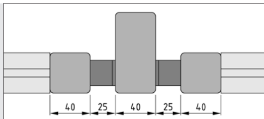
Aufhängung 8 in Verbindung mit Klemmprofil 8 40x40.
