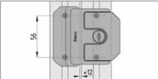
Bohrbild der Profile zur Anbringung des Türschlosses 6-8 Zn
