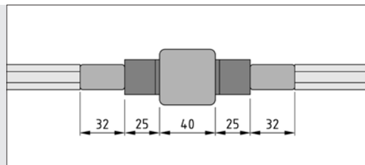
Aufhängung 8 in Verbindung mit Klemmprofil 8 32x18.
