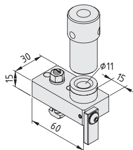
Bohrlehre 6, Klemmprofil 6 30x30
