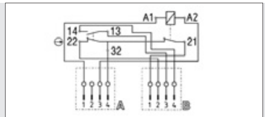
Anschluss-Schema: Sicherheits-Verriegelung kompakt
