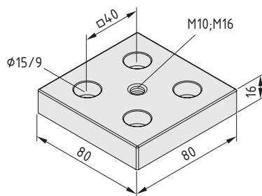
Transport- und Fußplatte X 8 80x80, M10
