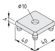
Fuß-Abdeckkappe 8 40x40 leicht
