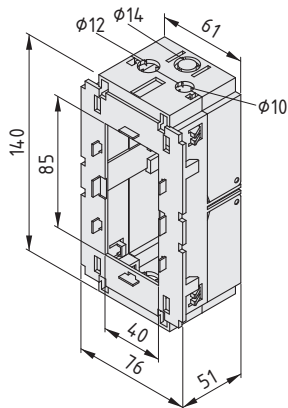
Einbaudose K76 M45 2-fach
