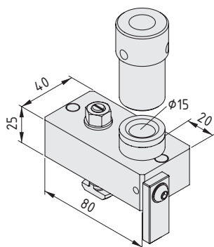
Bohrlehre 8, Klemmprofil 8 40x40
