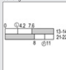
Darstellung der Schaltwege: Sicherheits-Endschalter kompakt
