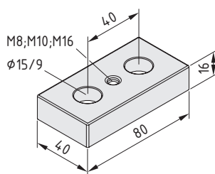
Transport- und Fußplatte X 8 80x40, M8
