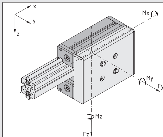
LRF 8 D10
