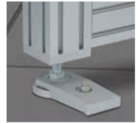
Klemmlaschen
