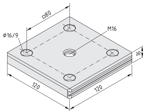
Transport- und Fußplatte 8 120x120, M16
