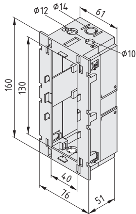
Einbaudose K76 M45 3-fach
