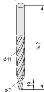
Stufenbohrer, Klemmprofil 6 30x30
