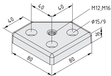
Transport- und Fußplatte 8 80x80-45°, M12
