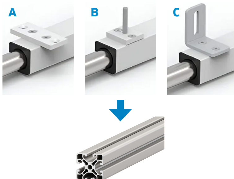
Montážní desky pro hliníkové profily (T-drážky)
